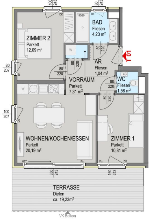
Grundriss Erdgeschoss
