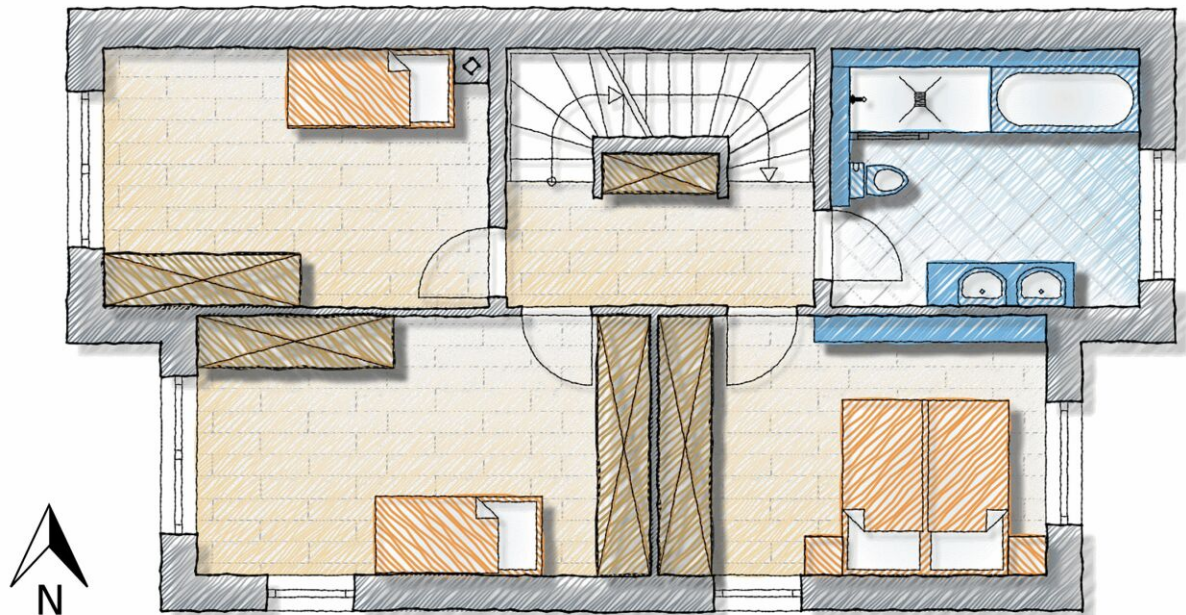
Grundriss Obergeschoss
