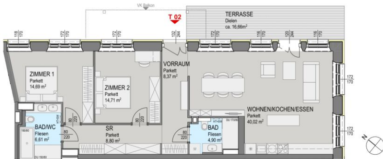
Grundriss Erdgeschoss
