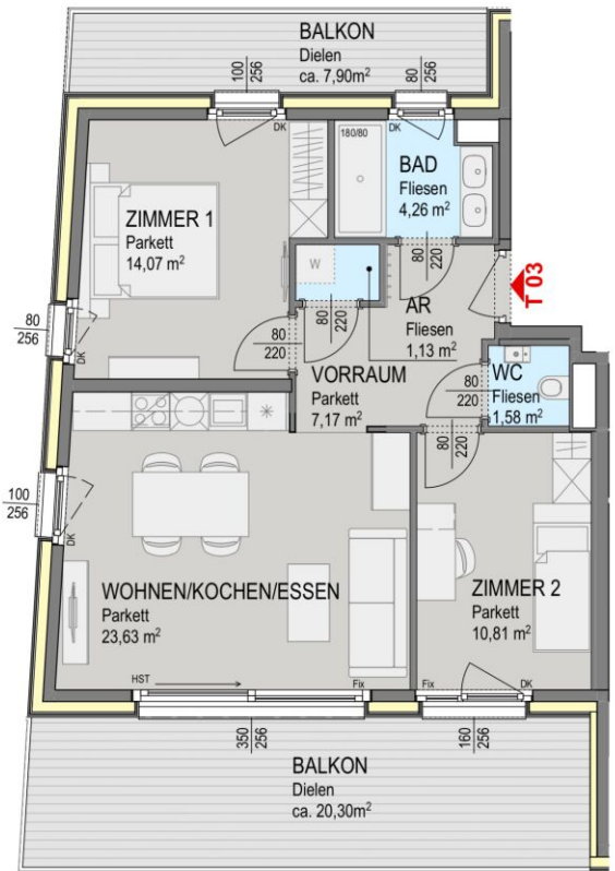
Grundriss Obergeschoss
