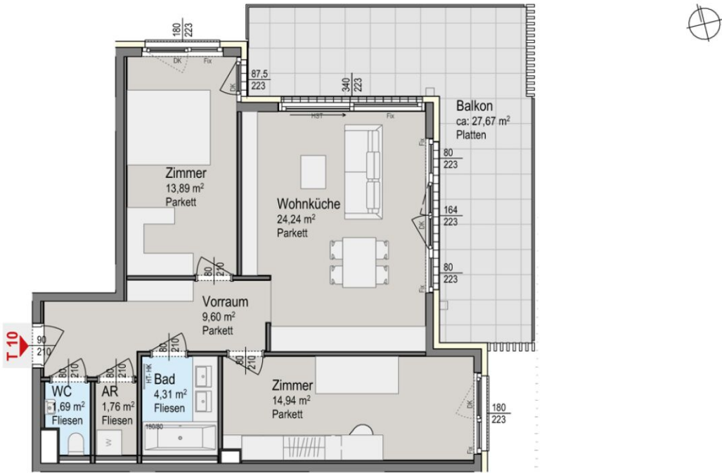
Grundriss 1. Obergeschoß
