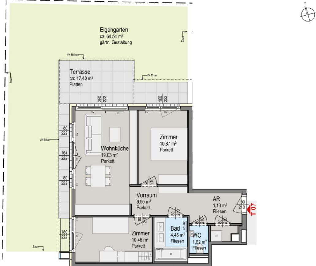
Grundriss Erdgeschoß
