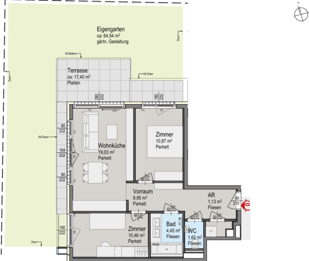
Grundriss Erdgeschoß
