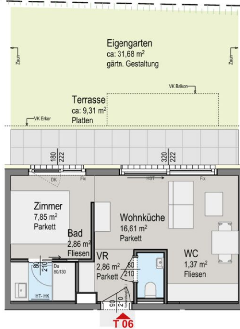
Grundriss Erdgeschoß
